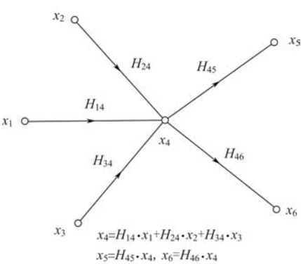
图 9-3 多输入输出混合节点
