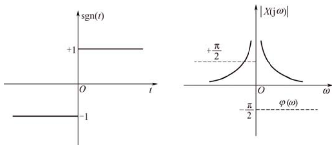
图 3-22 符号函数波形和频谱
