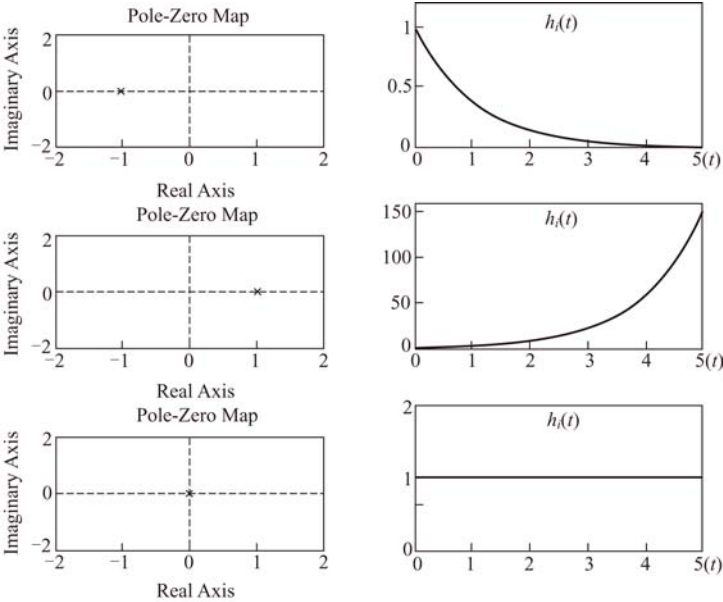
图 8-1 一阶实极点对应的的时间函数
