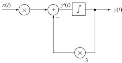
图 6-27 例 6-23 时域模拟框图
