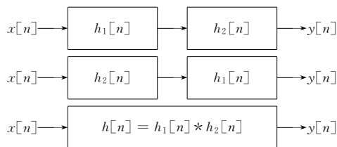
图 2-20 离散时间 LTI 系统的级联
