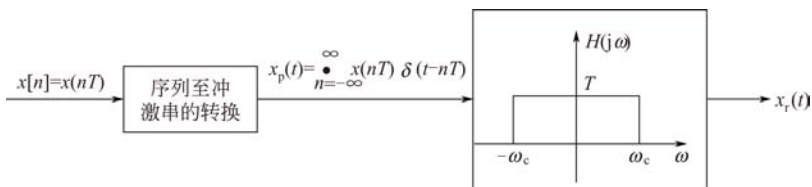
图 5-4 恢复系统
