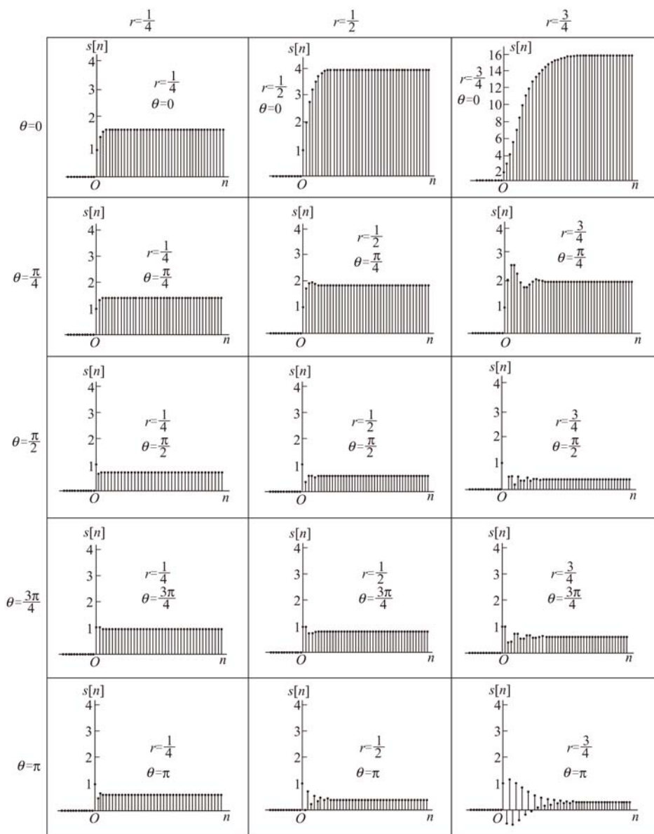
图 8-17 由方程式(8-65)表示的二阶系统的单位阶跃响应
