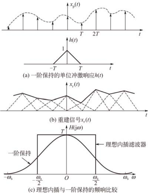
图 5-11 线性内插（一阶保持）
