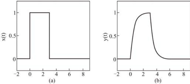
图 3-27 RC 低通网络对矩形脉冲的响应, E=1.0, T=3.0
