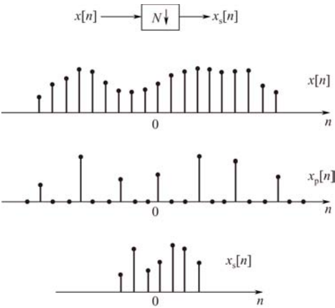
图 5-18 信号的抽取
