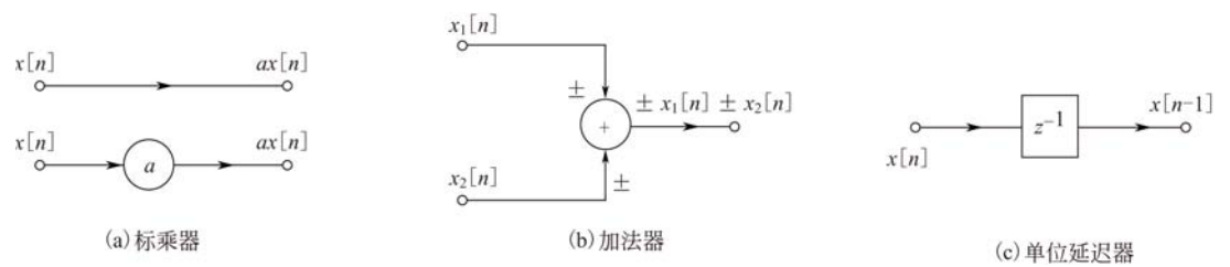
图 7-9 离散系统的三个基本运算单元
