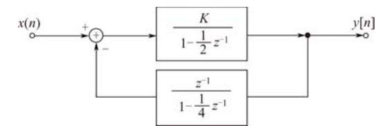
图 8-31 例 8-11 离散时间反馈系统
