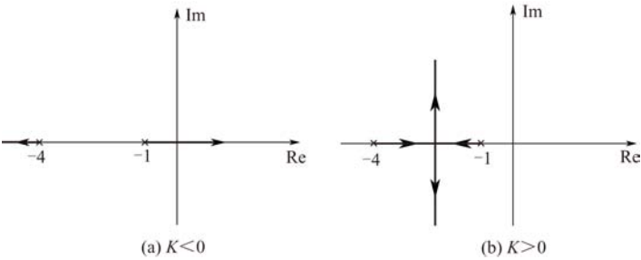
图 8-28 例 8-9 的根轨迹
