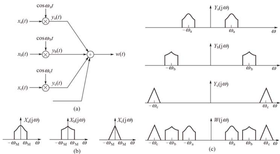
图 5-36 频分多路复用
