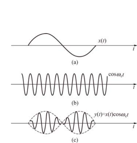
图 5-32 DSB 调制波形
