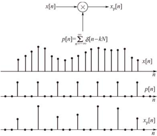
图 5-15 离散时间脉冲串采样
