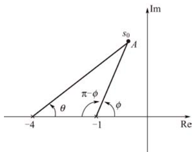
图 8-27 求满足角判据的几何方法
