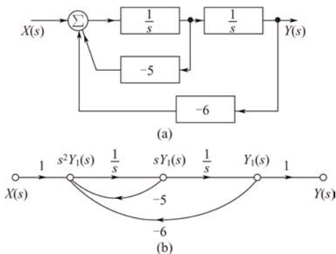
图 9-1 系统的模拟框图和信号流图表示
