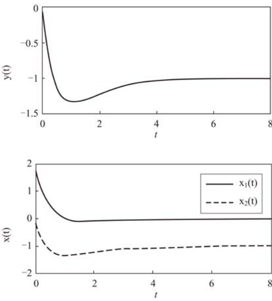
图 9-21 例 9-27 输出变量和状态变量响应曲线
