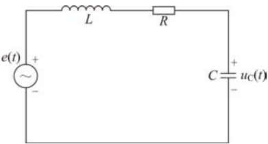
图 8-13 RLC 串联回路
