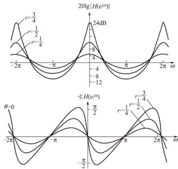
图 8-18 由方程式(8-65) 所描述的二阶系统的幅频响应与相频响应
