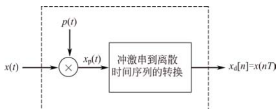
图 5-25 采样系统的等效模型
