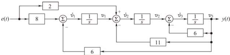
图 9-16 可观规范型
