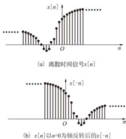
图 1-53 离散信号的反褶
