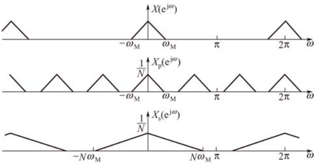
图 5-19 抽取的频域关系
