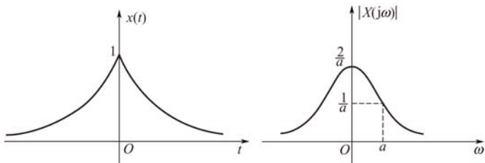
图 3-12 双边指数信号的波形及频谱
