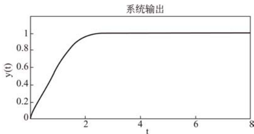
图 6-33 输出 y(t) , 例 6-30 图
