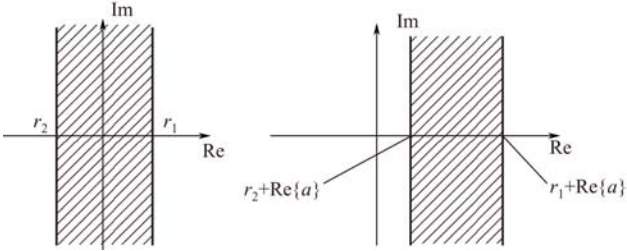
图 6-13 S 域平移的图解说明
