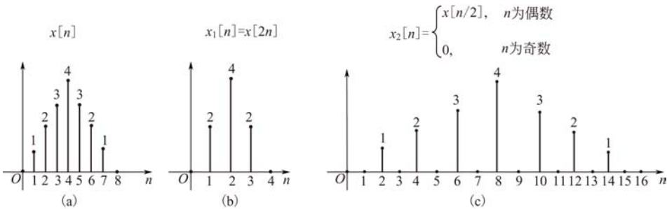
图 1-57 离散时间序列抽取和内插过程
