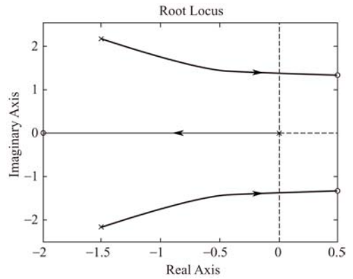
图 8-44 例 8-20 的根轨迹
