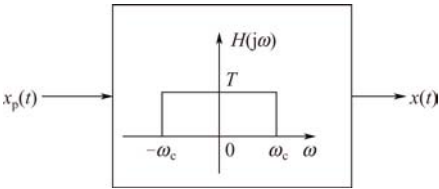
图 5-3 用于恢复的低通滤波器
