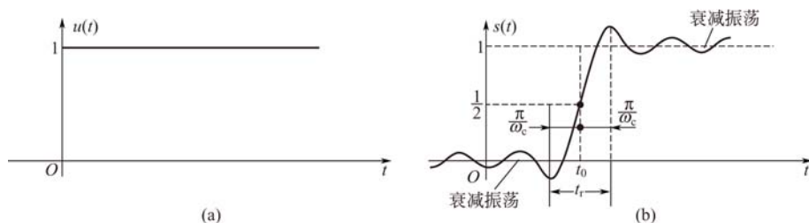
图 3-32 理想低通滤波器的阶跃响应
