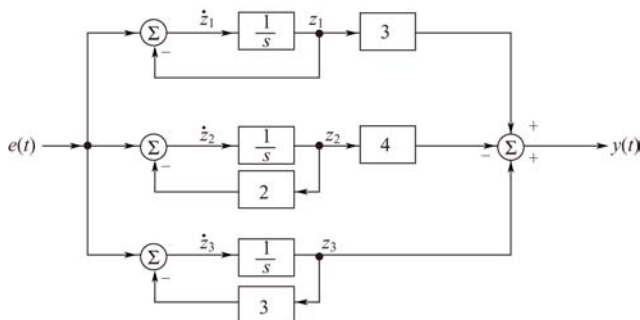
图 9-14 并联实现
