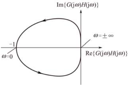
图 8-39 例 8-15 的奈奎斯特图
