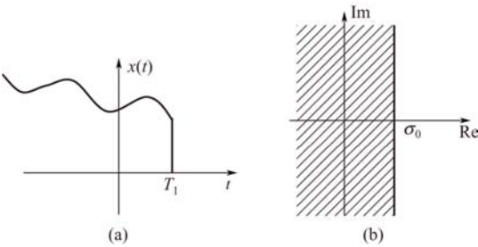
图 6-8 左边信号及其收敛域
