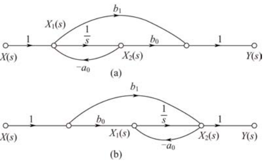
图 9-5 信号流图的转置
