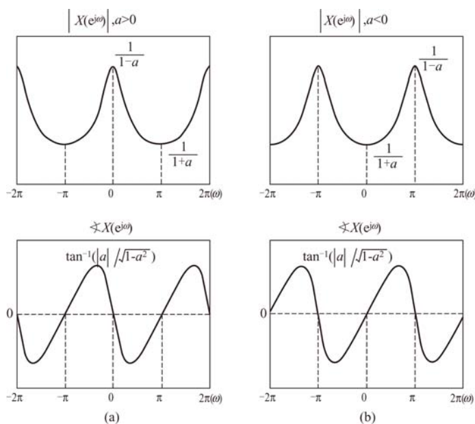
图 4-5 单边指数衰减信号的幅度谱与相位谱
