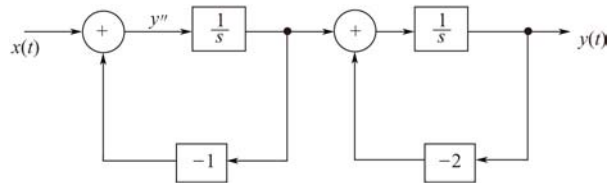
(b) 例6-25串联型图
