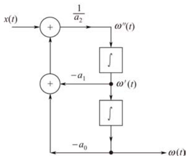
图 2-26 式(2-94) 所描述系统的模拟框图
