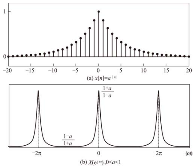
图 4-6 双边指数衰减信号及其频谱
