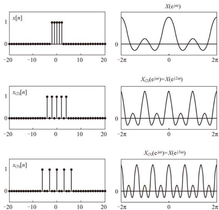
图 4-13 离散时间情况下时域与频域的相反关系：当 k 增加时， x_{(k)}[n] 在时域上拉开，而其傅里叶变换则在频域上压缩
