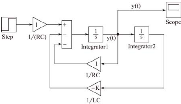
图 2-39 例 2-25 中 LC 并联电路的 Simulink 仿真框图
