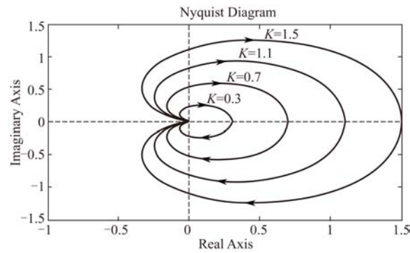
图 8-43 例 8-19 的奈奎斯特图
