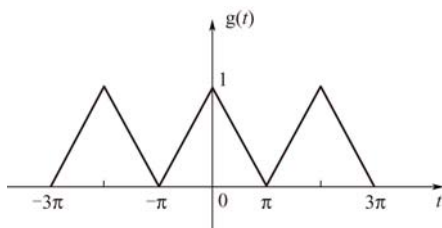
图 4-15 周期三角脉冲信号
