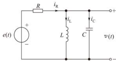
图 2-37 例 2-25 所讨论的 LC 并联电路
