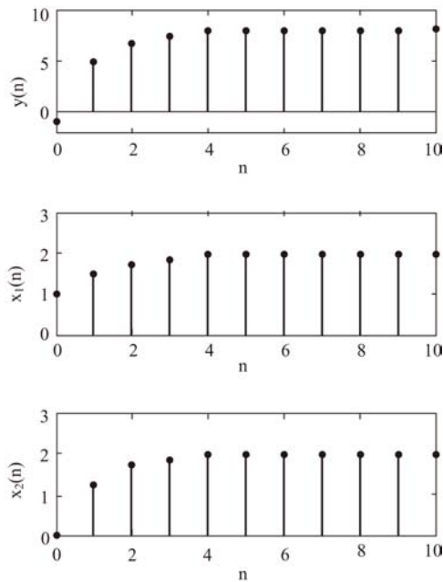
图 9-22 例 9-29 输出变量和状态变量响应曲线
