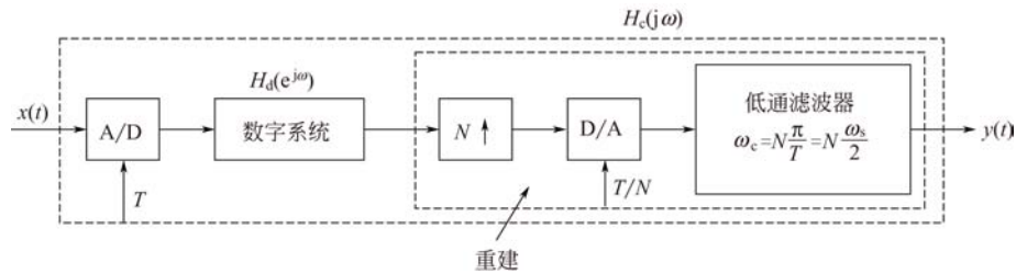
图 5-28 带限连续时间信号的数字化处理
