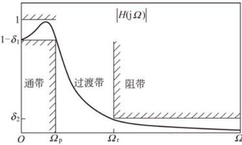
图 8-19 低通滤波器的幅频特性
