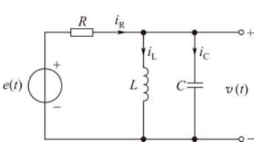
图 2-22 LC 并联电路
