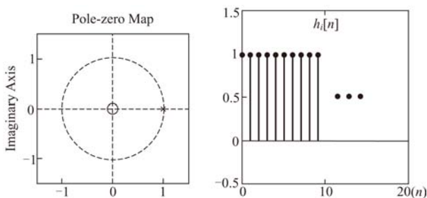
图 8-5 极点为 +1 及其对应的时间信号
