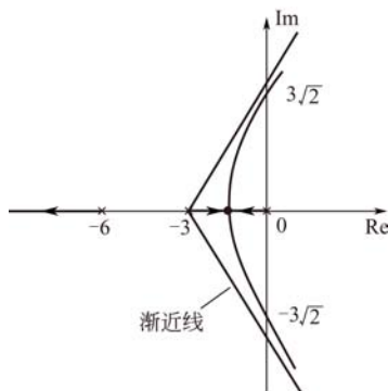
图 8-33 例 8-12 的根轨迹
