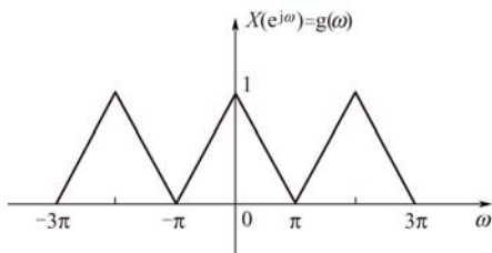
图 4-16 x[n] = \frac{1}{2} \text{Sa}^2\left(\frac{\pi n}{2}\right) 的傅里叶变换
