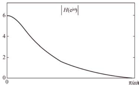
图 4-23 例 4-20 系统的幅度响应
