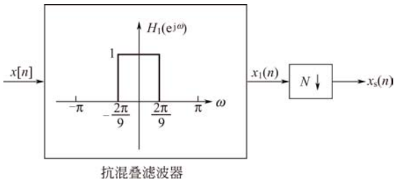
图 5-21 信号的最大抽取
