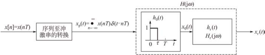
图 5-9 零阶保持的恢复系统
