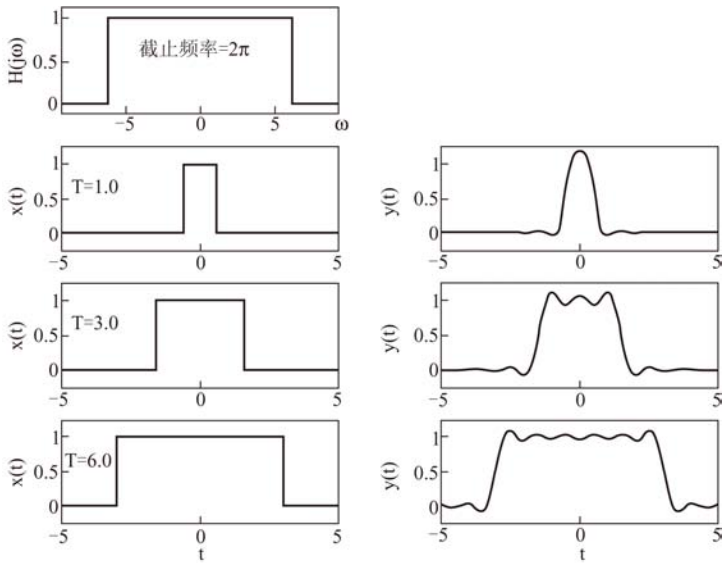
图 3-33 理想低通滤波器对矩形脉冲的响应
