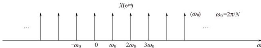
(b) 离散时间周期冲激串的频谱
