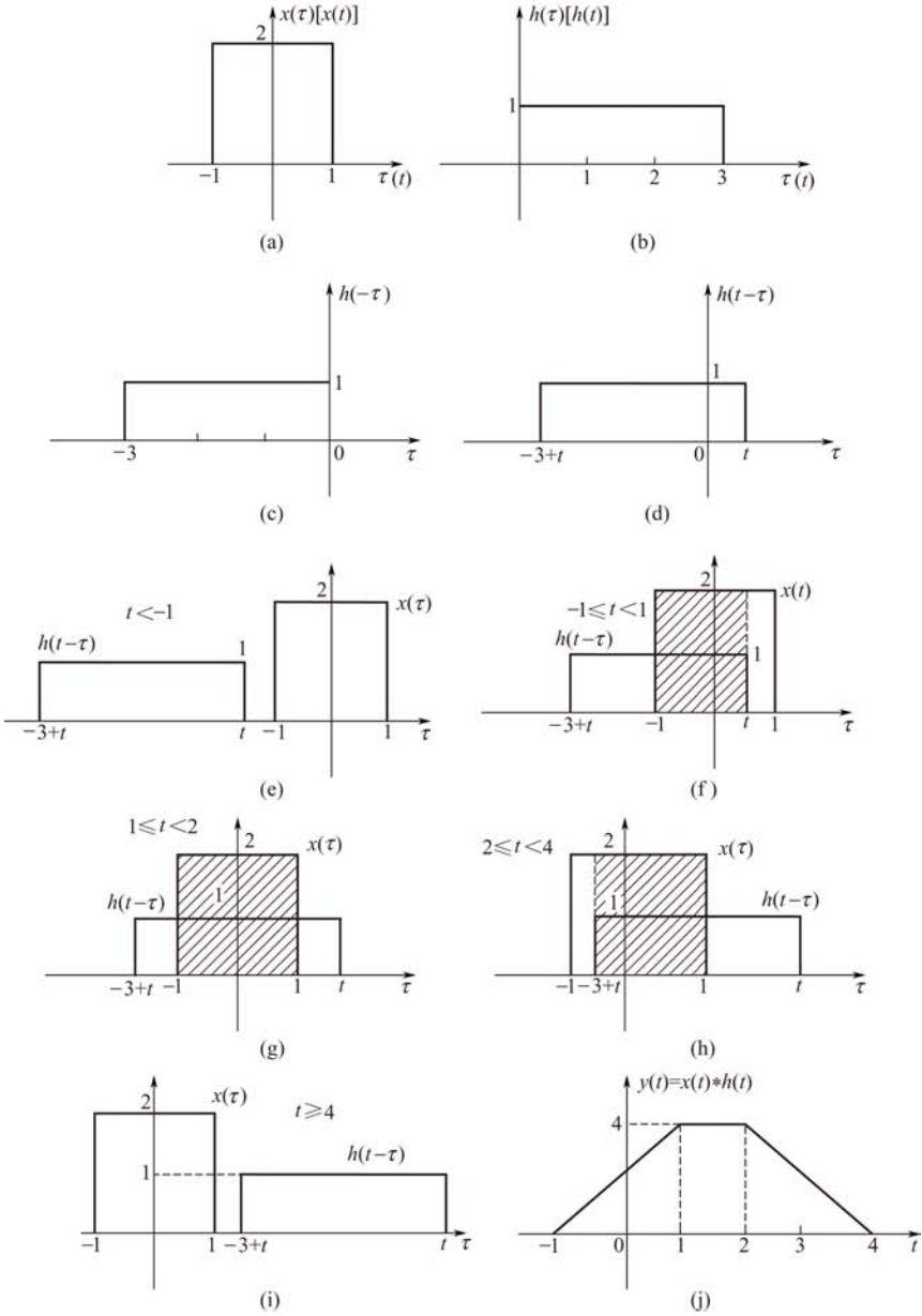
图 2-8 例 2-2 卷积的图解示意图
