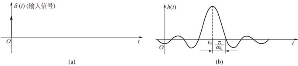
图 3-31 理想低通滤波器的冲激响应
