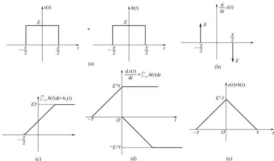
图 2-16 用卷积微分、积分性质计算卷积
