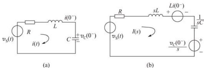
图 6-25 RLC 电路 S 域模型
