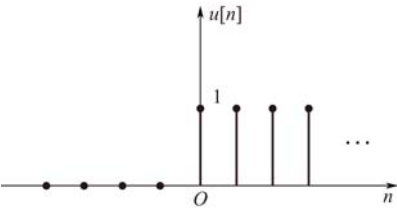
图 1-36 u[n] 信号
