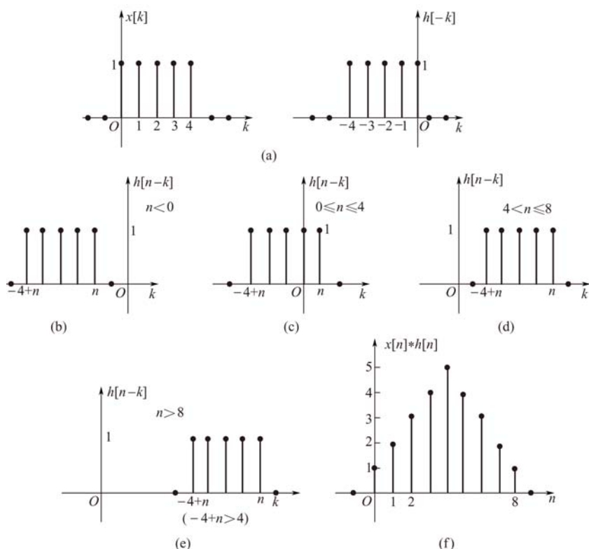
图 2-19 例 2-7 图解说明
