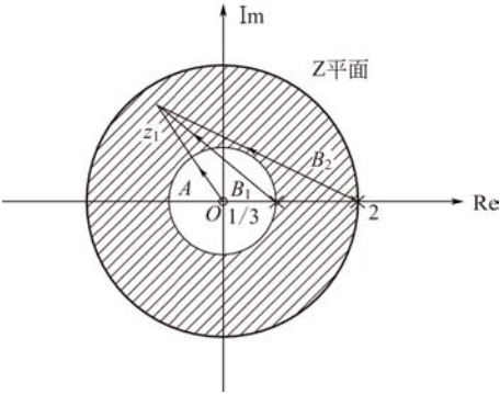
图 7-7 零极点矢量
