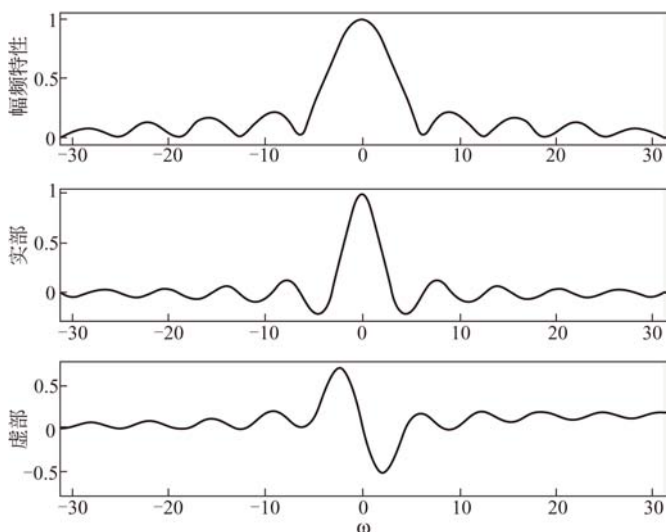
图 3-17 方波的频谱
