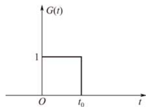
图 1-21 矩形脉冲
