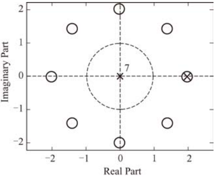
图 7-14 例 7-30 零极点图
