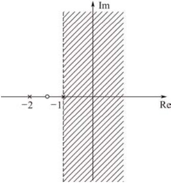
图 6-4 例 6-3 的收敛域
