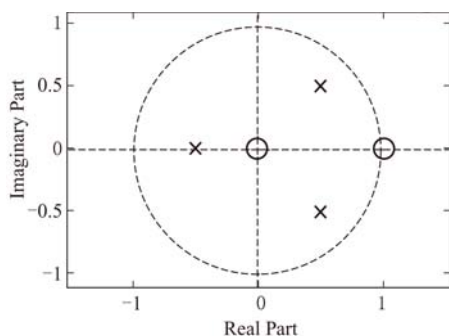
图 7-15 例 7-31 零极点图
