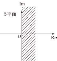
图 6-12 例 6-6 的 ROC
