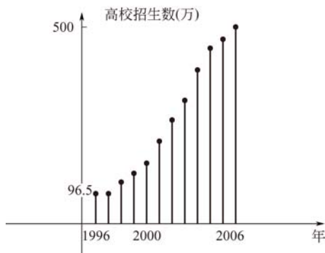
图 1-4 中国近十年高校招生人数离散信号
