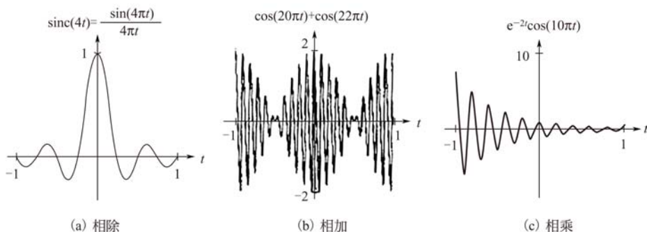
图 1-45 信号的组合
