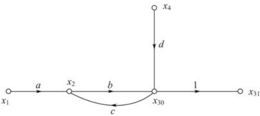
图 9-4 将一个节点分成两个节点
