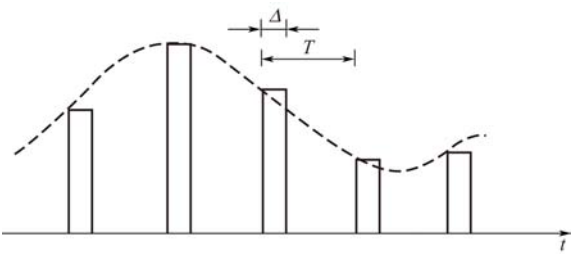
图 5-41 一路平顶采样形式传输的波形，图中虚线代表信号 x(t)
