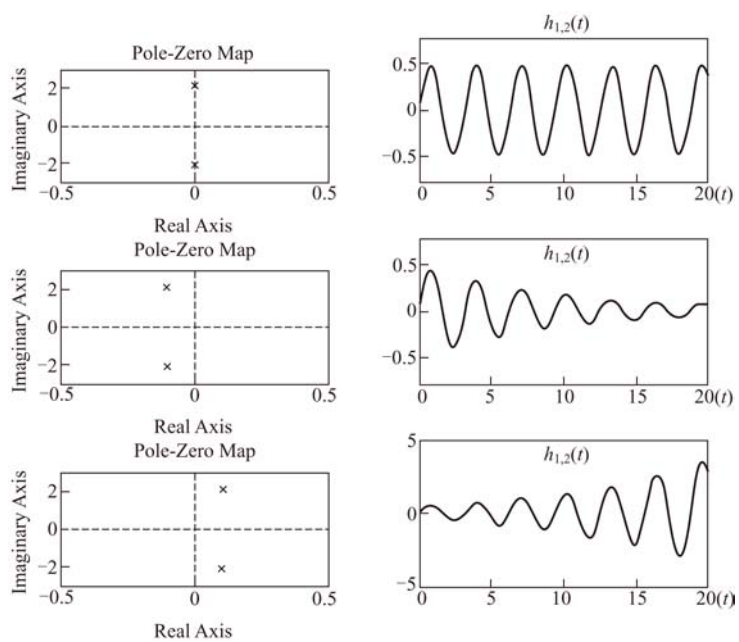
图 8-2 一阶共轭复极点对应的的时间函数
