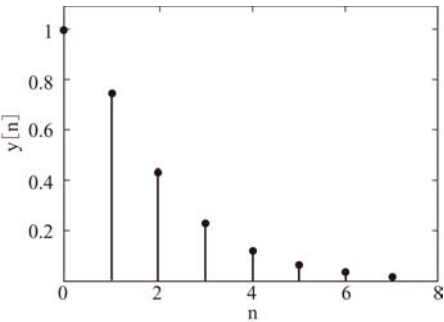
图 7-13 例 7-29 零状态响应波形
