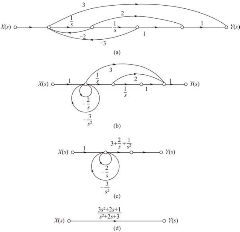
图 9-7 流图的化简示例
