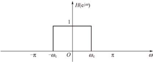
图 4-18 离散时间理想低通滤波器的频率响应
