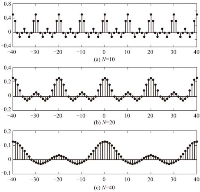
图 4-2 例 4-2 周期方波的傅里叶级数系数
