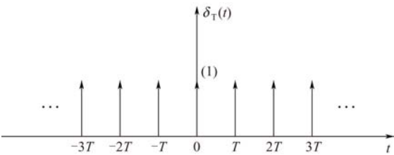
图 1-30 单位连续冲激串信号波形
