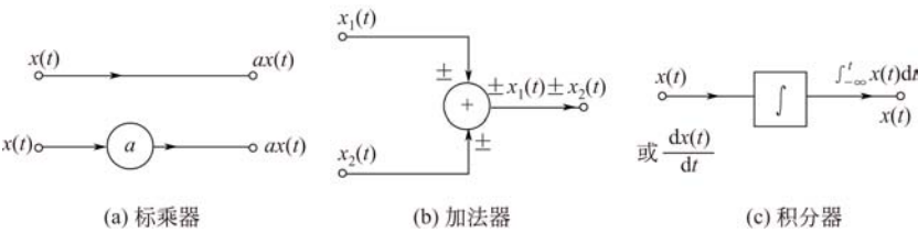
图 2-25 三种基本运算器的模型符号
