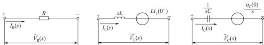
图 6-23 元件的电压降与电流关系的 S 域模型（回路分析）
