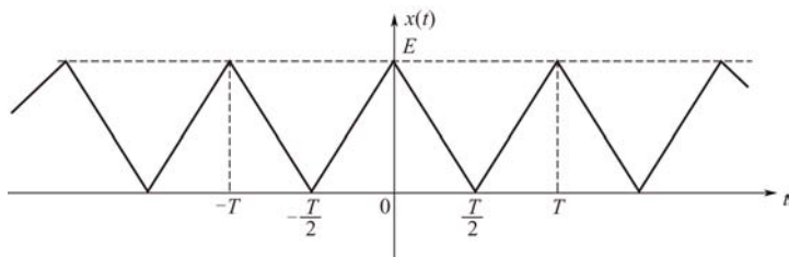
图 3-5 周期三角脉冲信号的波形
