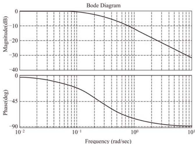
图 8-41 例 8-17 的波特图
