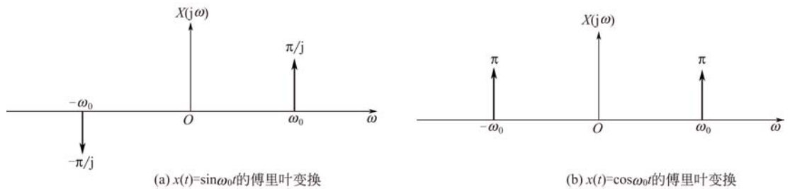
图 3-19 正弦和余弦信号的频谱
