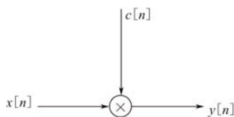
图 5-44 离散时间幅度调制
