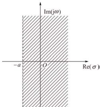
图 6-1 X_1(s) 的收敛域
