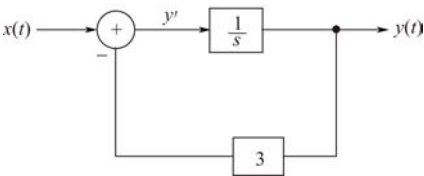
图 6-28 例 6-23 S 域模拟框图
