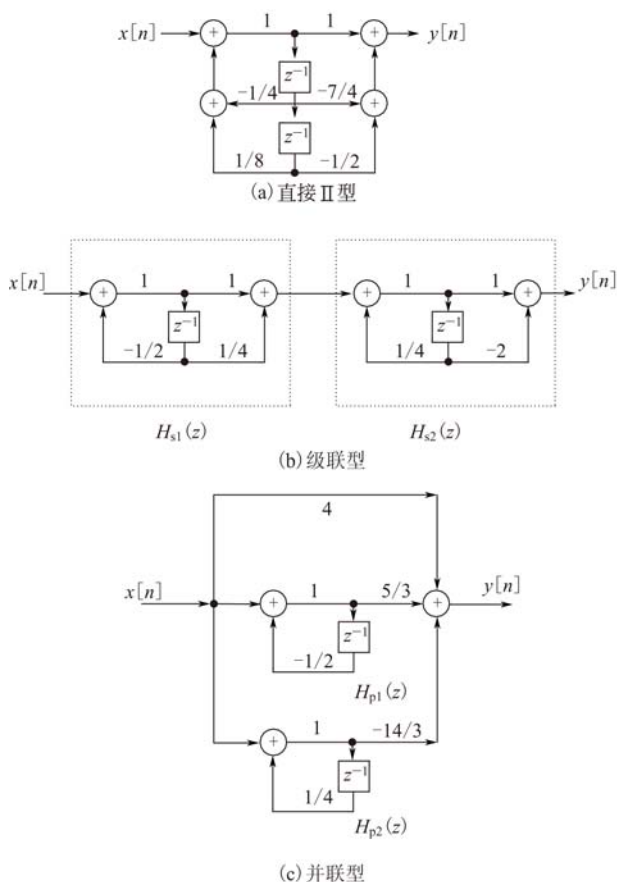
图 7-12 例 7-25 系统的 Z 域框图表示
