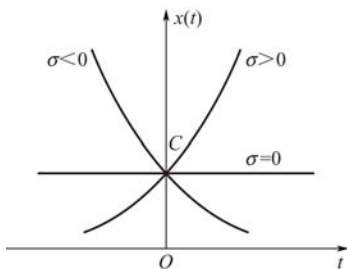
图 1-11 连续时间实指数信号
