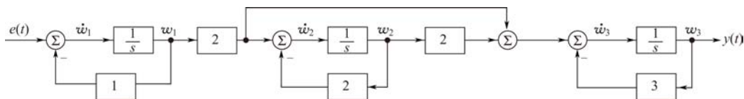
图 9-13 串联实现
