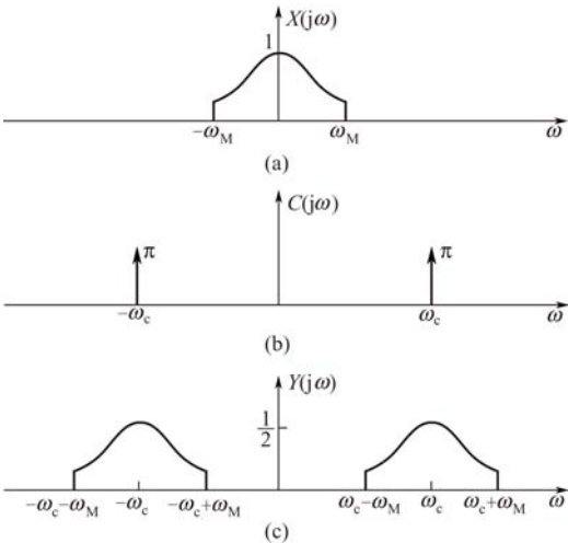
图 5-33 DSB 调制的频谱说明
