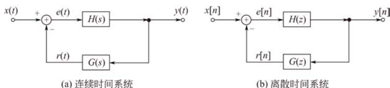
图 8-25 基本 LTI 反馈系统结构
