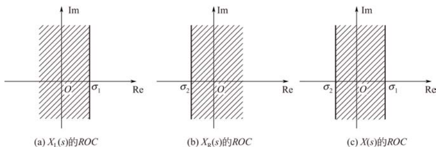
图 6-10 双边信号的拉氏变换收敛域
