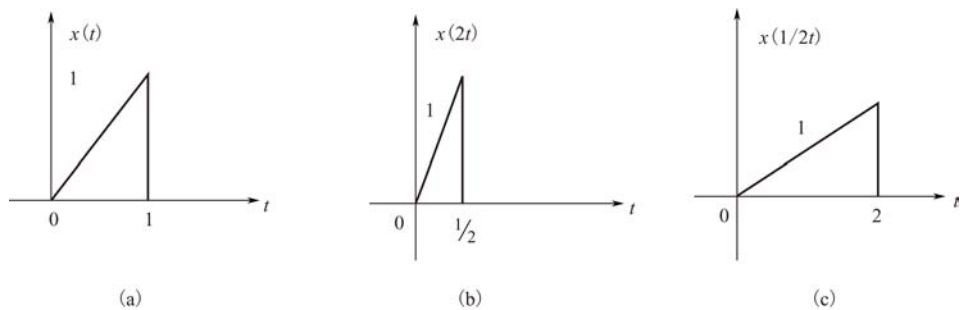
图 1-54 信号的尺度变换
