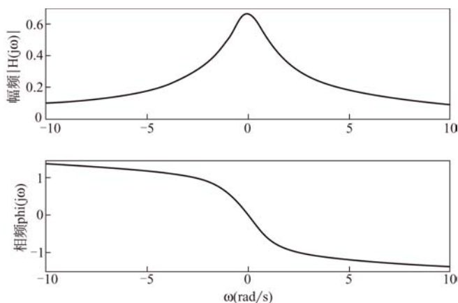
图 3-25 例 3-17 频率响应的幅频特性和相频特性
