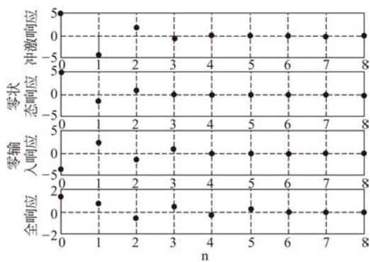
图 2-34 例 2-22 的运行结果图
