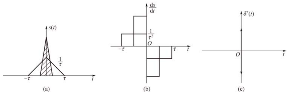
图 1-29 冲激偶信号
