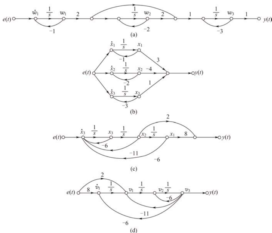
图 9-17 用信号流图来表示系统
