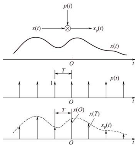
图 5-1 冲激串采样
