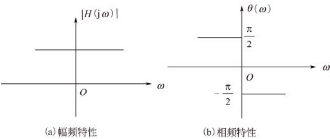
图 5-43 理想的 \frac{\pi}{2} 移相器
