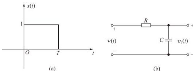
图 3-34 RC 低通网络
