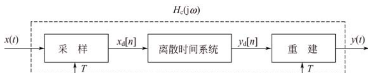
图 5-24 连续时间信号的离散时间处理, 其中 x_d[n] = x(nT) , y_d[n] = y(nT)
