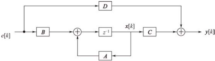
图 9-18 离散系统状态变量分析的示意图
