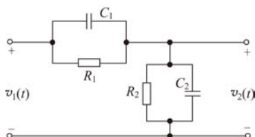
图 3-29 无失真传输系统电路图 (当 R_1 C_1 = R_2 C_2 时)
