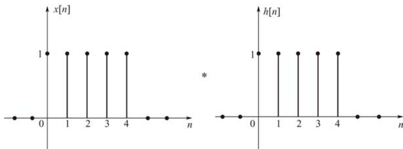
图 2-18 例 2-7 中 x[n] 和 h[n] 的波形
