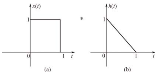
图 2-6 x(t) 和 h(t) 的波形
