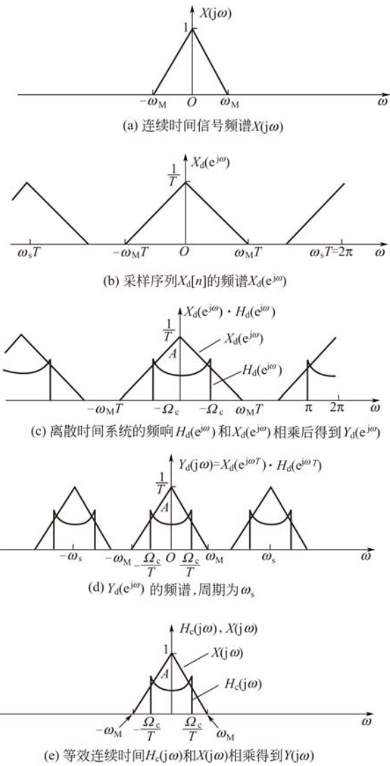
图 5-27 系统的频域说明
