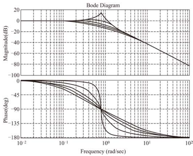
图 8-42 例 8-18 的波特图
