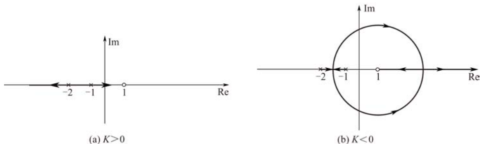
图 8-30 例 8-10 的根轨迹
