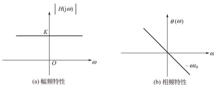
图 3-28 无失真传输系统的频率响应特性
