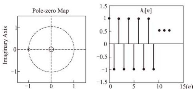
图 8-6 极点为 -1 及其对应的时间信号
