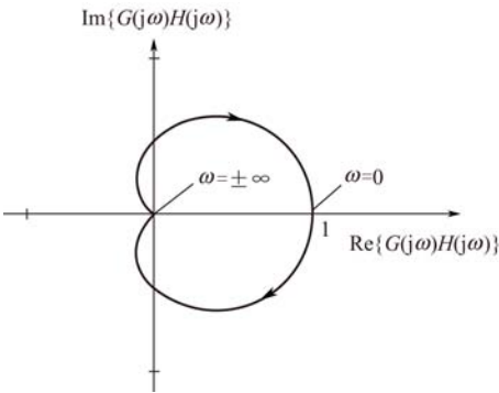
图 8-38 例 8-14 的 G(j\omega)H(j\omega) 的奈奎斯特图
