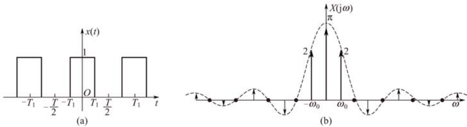
图 3-18 周期对称方波的傅里叶变换 ( T=4T_1 )
