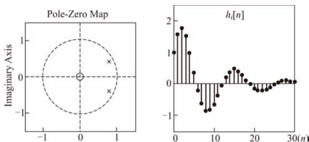
图 8-4 单位圆内一阶共轭复极点及其对应的时间信号
