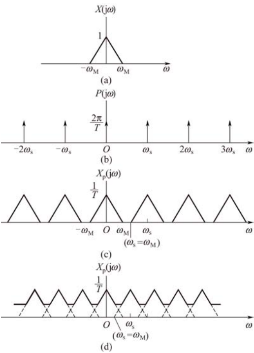
图 5-2 时域采样的各信号的频谱
