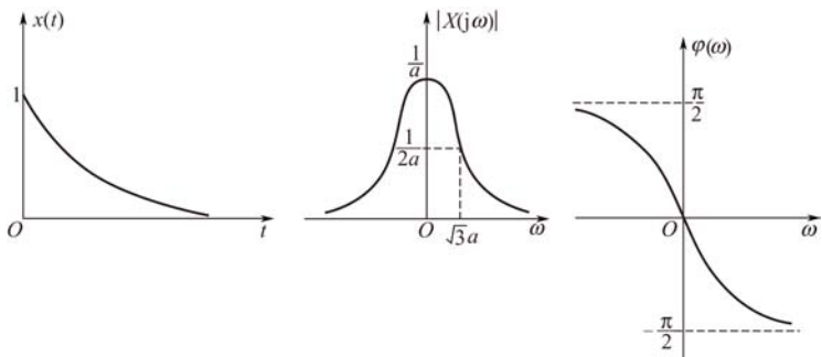
图 3-11 单边指数信号的波形及频谱
