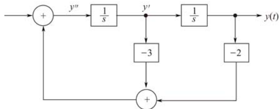
(a) 例6-25直接型图
