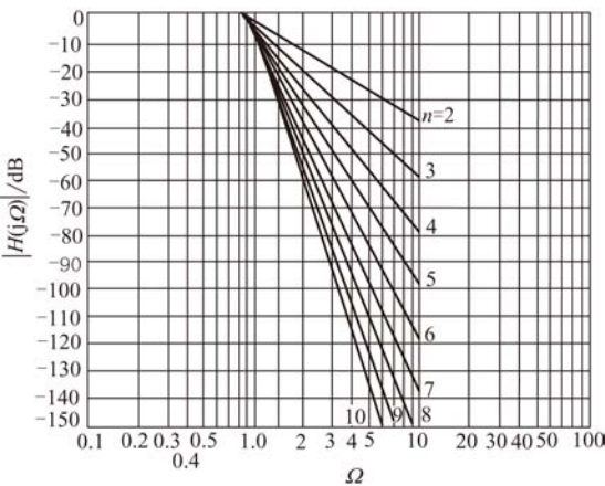
图 8-23 巴特沃思滤波器的幅频特性（波特图）
