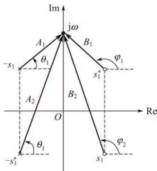
图 8-10 二阶全通系统的零极点矢量图
