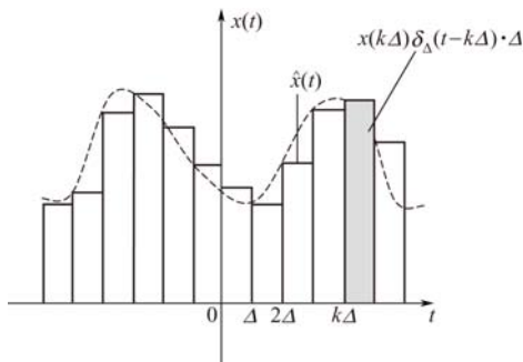
图 2-4 用矩形脉冲逼近 x(t)
