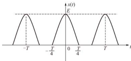
图 3-6 周期半波余弦信号波形
