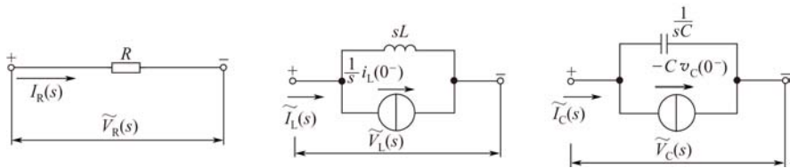
图 6-24 S 域元件模型（节点分析）
