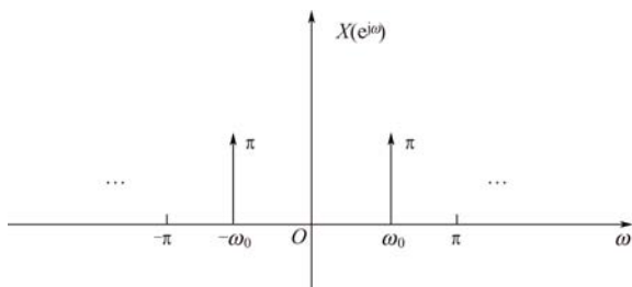
图 4-10 x[n] = \cos\omega_0 n 的离散时间傅里叶变换
