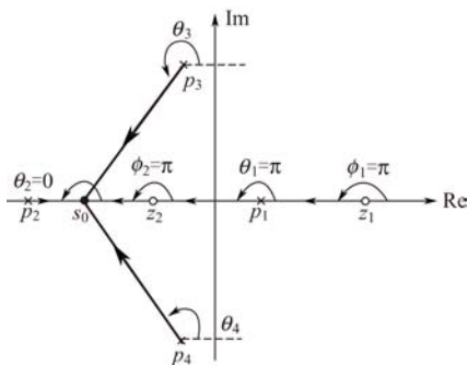
图 8-29 检验实轴上的根轨迹
