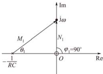
图 6-21 高通滤波器的零极点图
