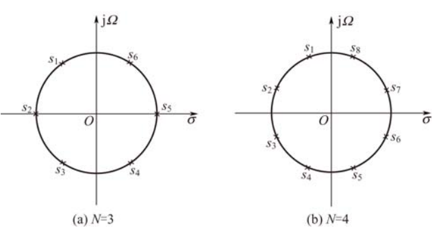
图 8-22 巴特沃思低通滤波器 |H(s)|^2 的极点分布
