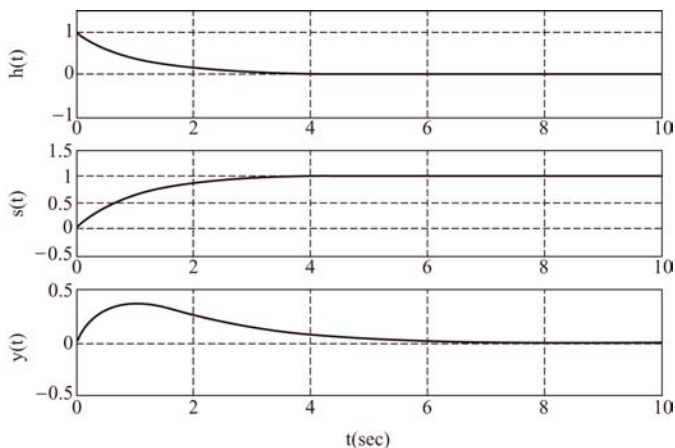
图 2-32 例 2-20 的运行结果图
