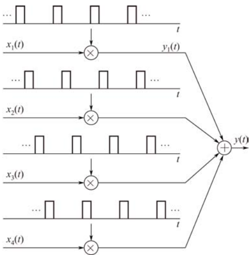
图 5-40 时分复用
