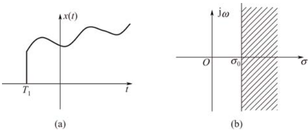
图 6-7 右边信号及其收敛域
