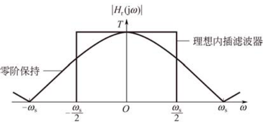
图 5-8 零阶保持和理想滤波器的频响特性
