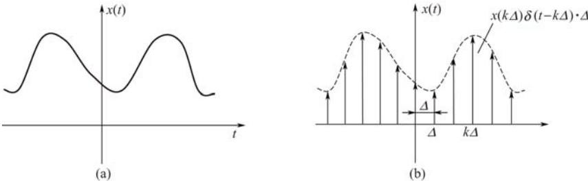
图 2-1 用移位冲激函数逼近 x(t)
