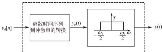
图 5-26 重建系统的等效模型
