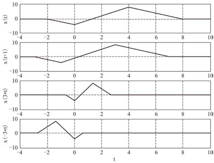
图 1-56 变换函数的波形 (例 1-11 图)
