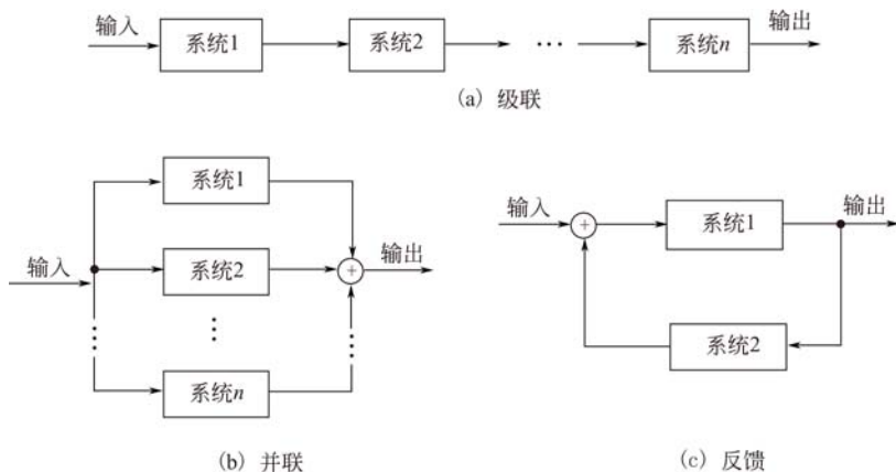
图 1-59 系统的互联
