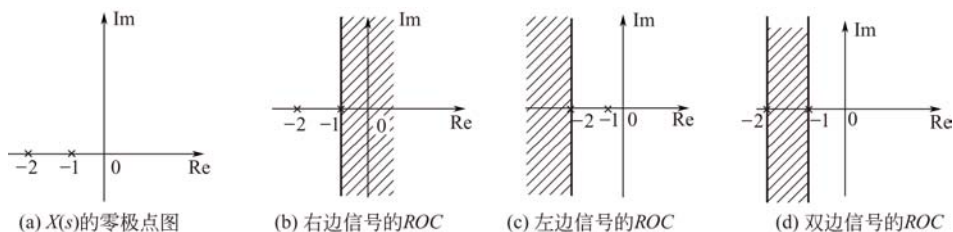
图 6-11 例 6-4 信号拉氏变换 X(s) 的收敛域
