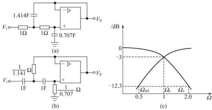
图 8-24 低通与高通滤波器的幅频特性
