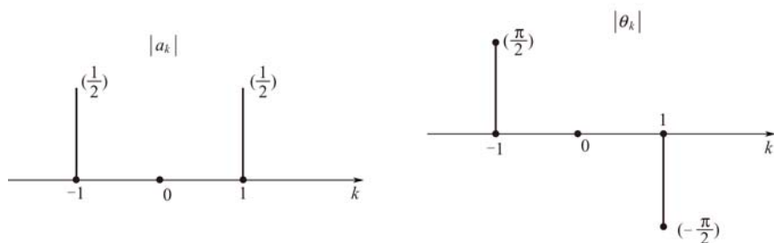
图 3-1 \sin\omega_0 t 信号的傅里叶级数系数的幅度和相位
