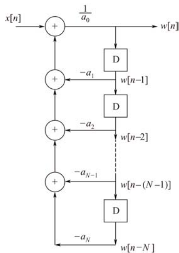
图 2-30 式(2-99) 所描述离散时间系统的模拟框图
