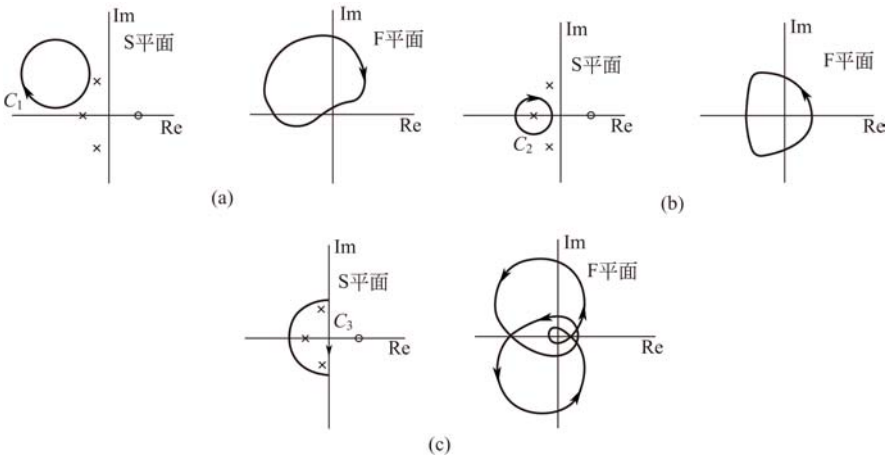
图 8-35 例 8-13 围线映射图
