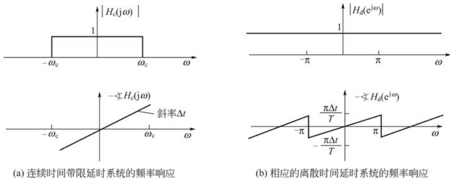
图 5-30 带限延时器的频率响应
