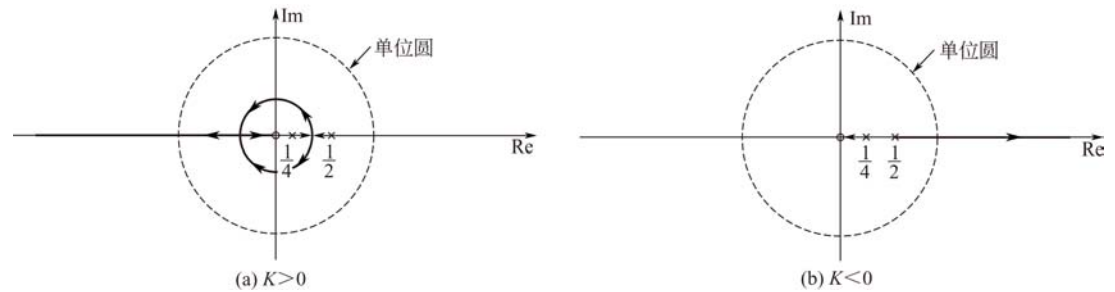
图 8-32 例 8-11 的根轨迹
