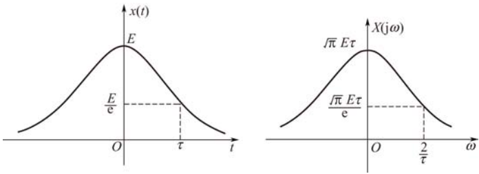
图 3-16 高斯脉冲信号的波形及频谱
