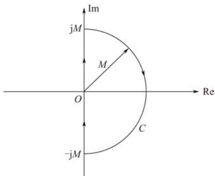
图 8-36 包括右半平面的半圆闭合围线, 当 M \rightarrow \infty 时, 该围线包括了整个右半平面
