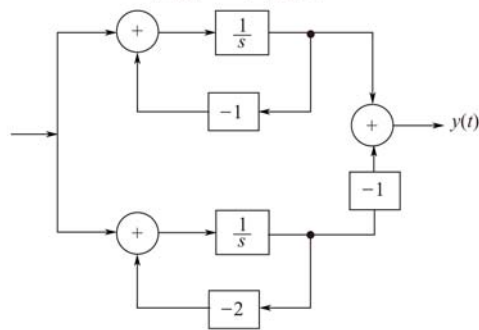
(c) 例6-25并联型图
