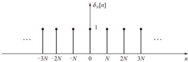
图 1-40 单位离散冲激串序列的波形
