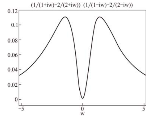
图 3-23 两相加指数信号的能量密度谱
