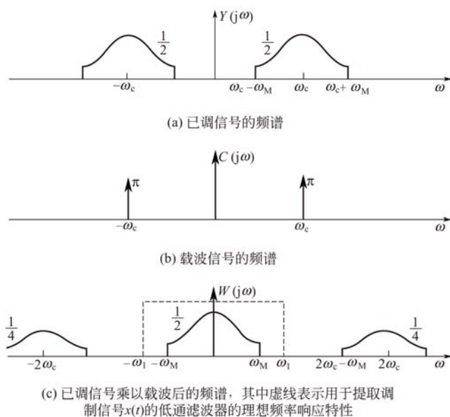
图 5-35 同步解调的频谱说明
