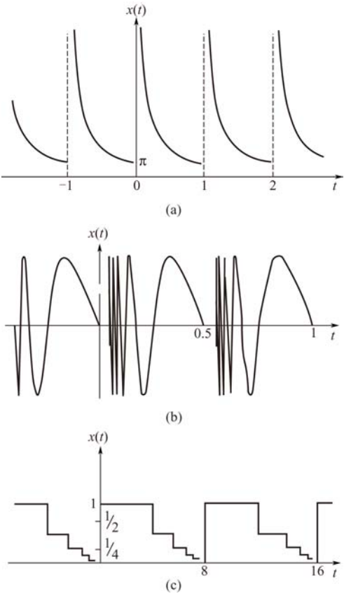
图 3-8 不满足狄里赫利条件的信号
