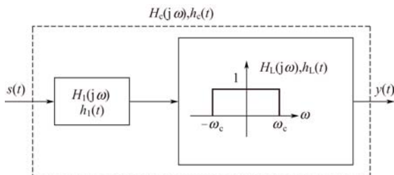
图 5-29 带限回波消除器
