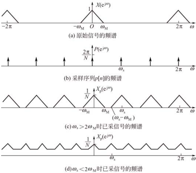
图 5-16 脉冲串采样后的频谱图
