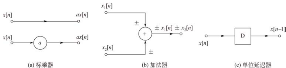
图 2-29 离散系统的三个基本运算单元
