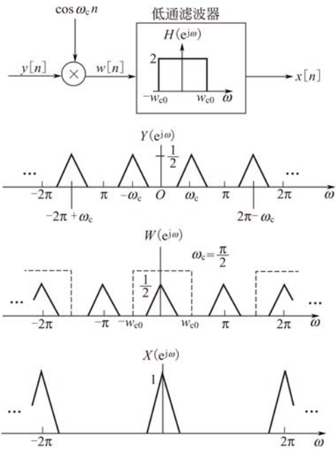
图 5-46 离散时间同步解调及其相关频谱说明 ( \omega_c = \frac{\pi}{2} )
