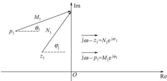
图 6-19 零点、极点矢量
