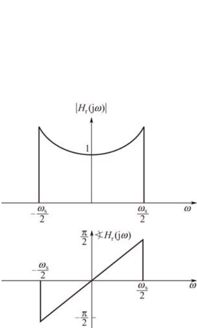
图 5-10 零阶保持输出信号的重建滤波器的模和相位特性
