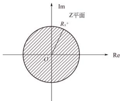
图 7-4 左边序列的 ROC
