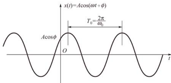
图 1-12 具有初始相位的正弦信号
