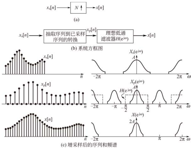
图 5-20 信号的增采样（内插）
