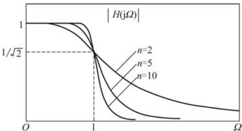
图 8-21 n = 2, 5, 10 时的巴特沃思滤波器的幅频特性
