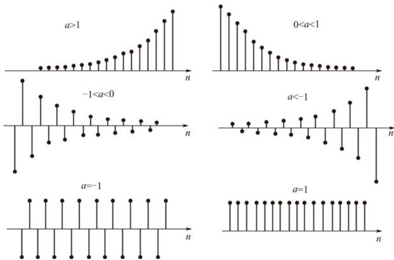
图 1-41 实指数序列
