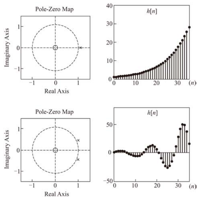
图 8-8 单位圆外的一阶实极点与共轭极点的时间信号
