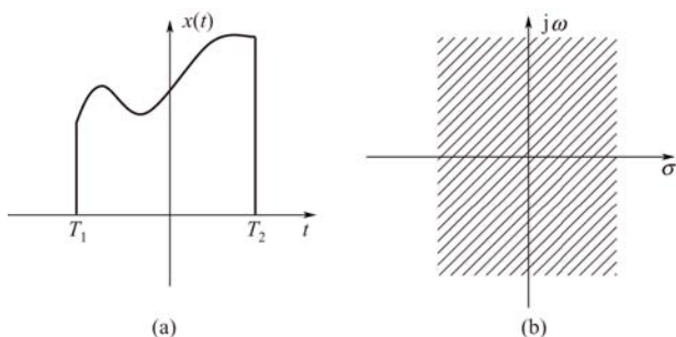
图 6-5 时限信号 x(t) 及其收敛域
