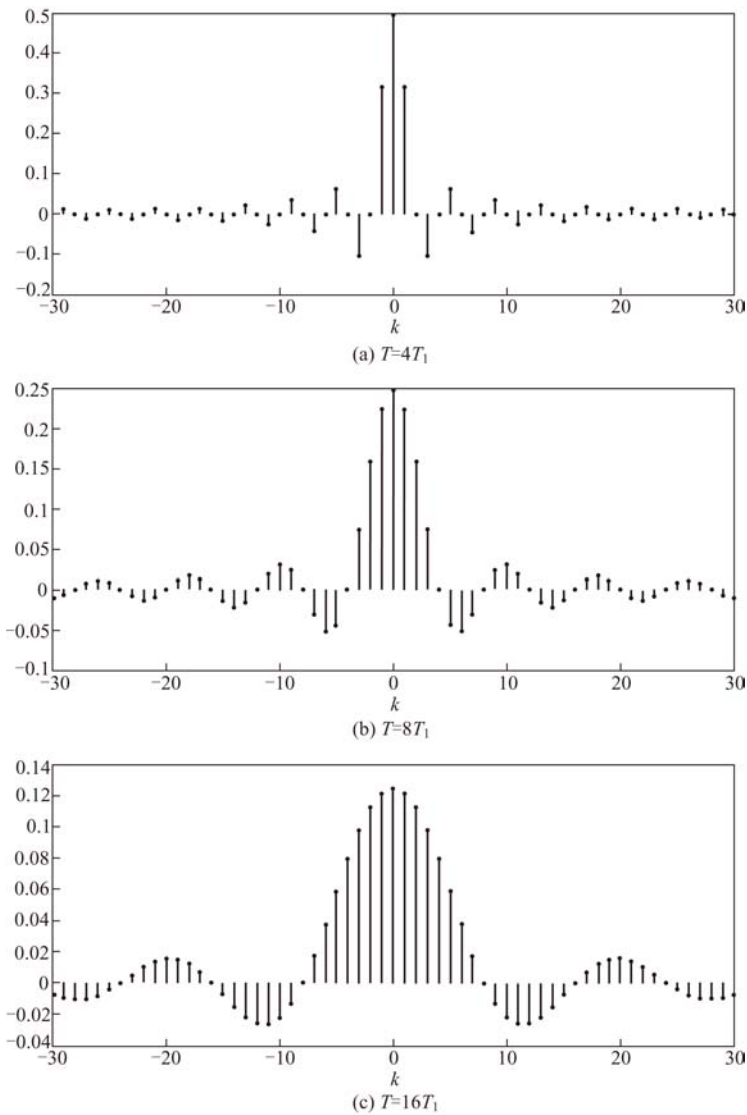
图 3-3 对于 T_1 固定和几个不同的 T 值时，周期方波傅里叶级数系数 a_k 的图 (a) T=4T_1 ；(b) T=8T_1 ；(c) T=16T_1 。周期逐渐增大， 其样本间隔 \omega_0 将随 T 的增加而减少
