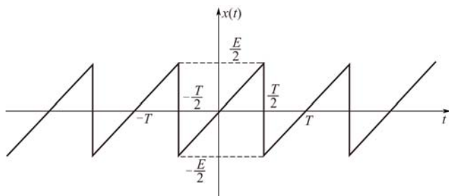
图 3-4 周期锯齿脉冲信号的波形
