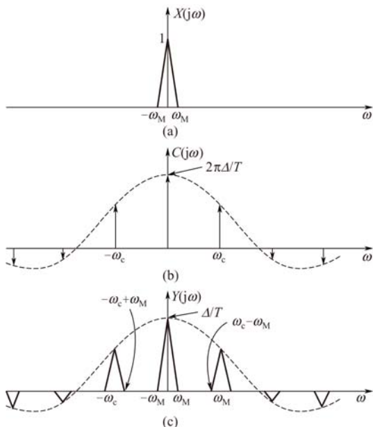
图 5-39 自然采样形式的脉冲幅度调制的频谱说明
