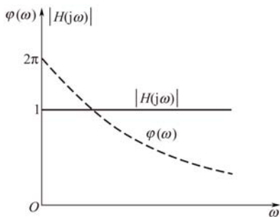
图 8-11 二阶全通系统的频率响应
