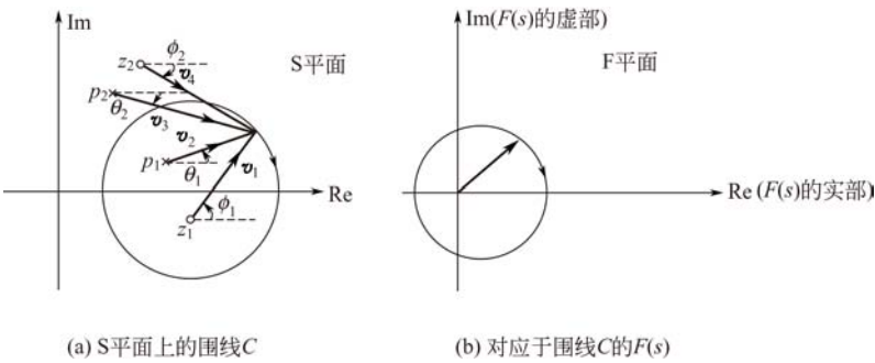
图 8-34 从 S 平面到 F 平面的围线映射
