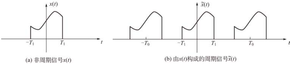
图 3-10 非周期信号的周期延拓
