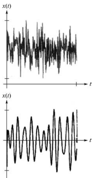
图 1-3 随机信号
