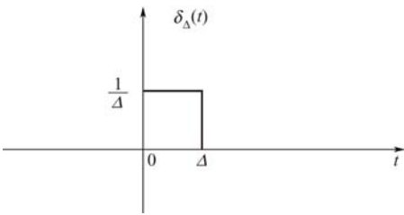
图 1-25 \delta_{\Delta}(t) 的波形
