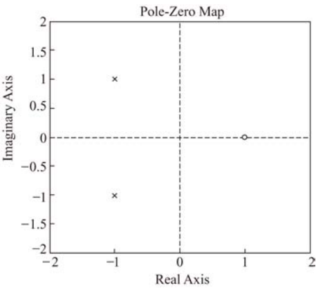
图 6-31 例 6-28 零极点图
