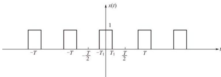
图 3-2 周期方波
