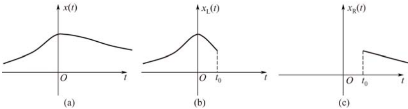
图 6-9 双边信号
