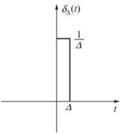
图 2-2 \delta_{\Delta}(t) 波形
