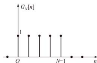
图 1-38 矩形序列
