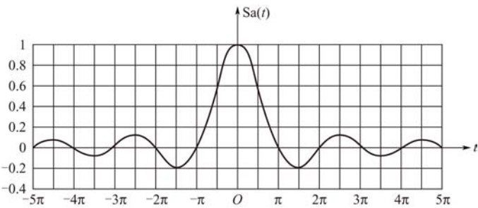
图 1-31 Sa(t) 波形
