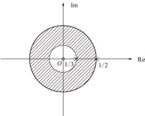
图 7-6 例 7-5 的 ROC
