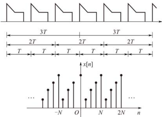
图 1-5 周期信号
