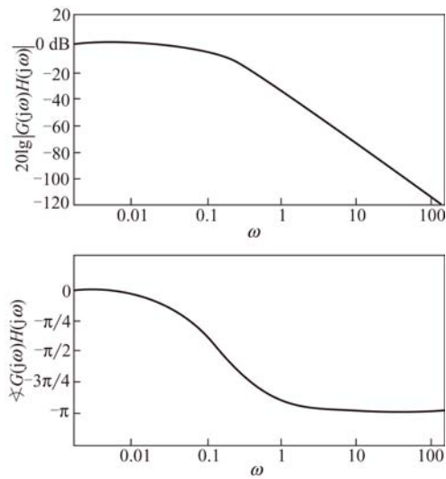
图 8-37 例 8-14 的 G(j\omega)H(j\omega) 的波特图
